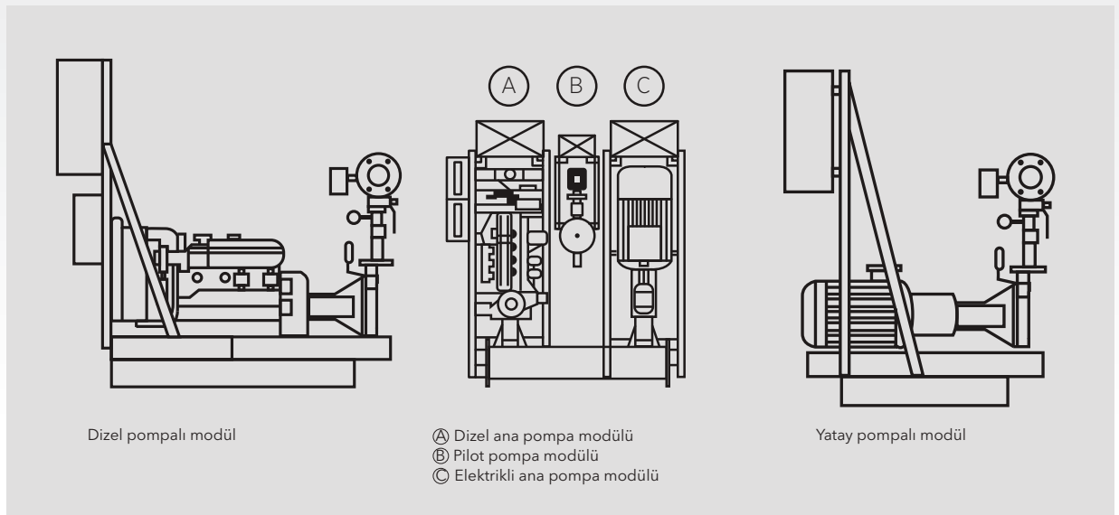
Şekil 1: Modüler Sistem
