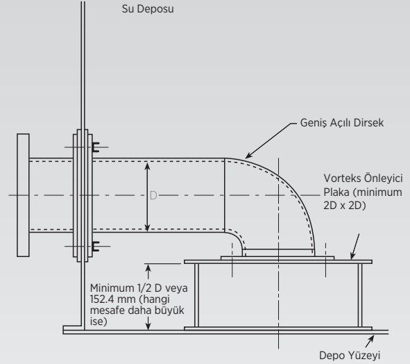
Şekil 3: Vorteks Plakası Ölçüleri
