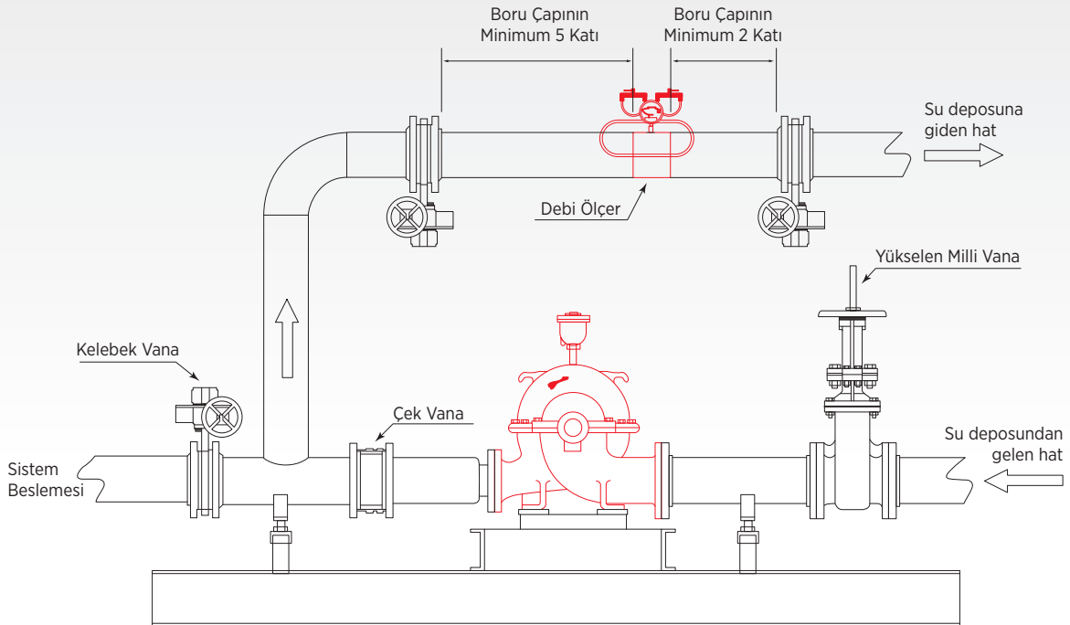
Şekil 4: Debimetre Bağlantı Şeması
